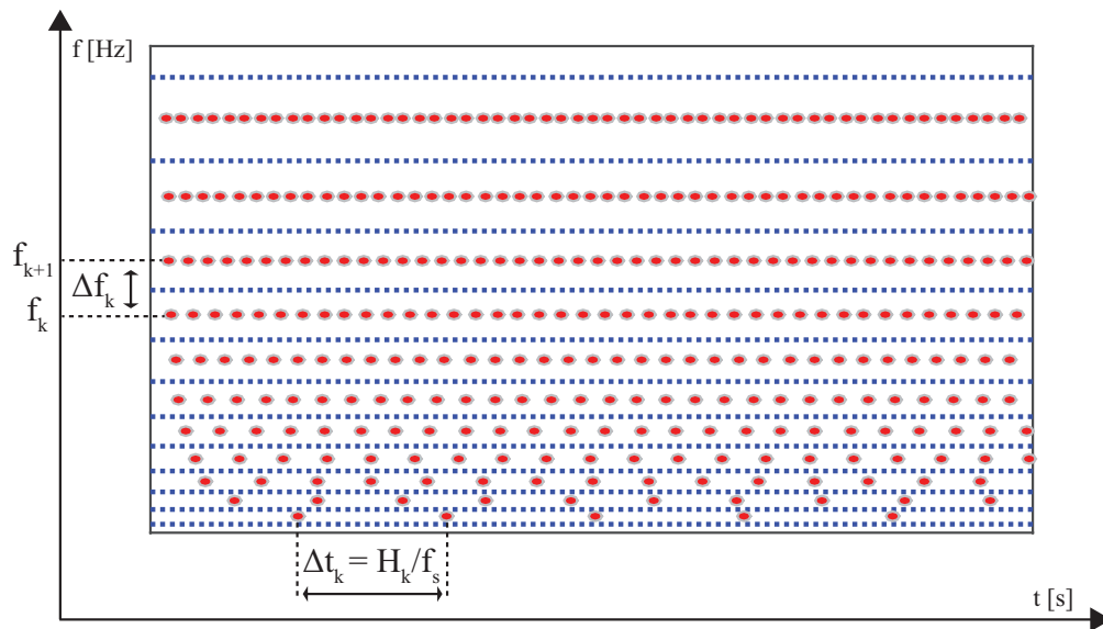
(b) CQT
